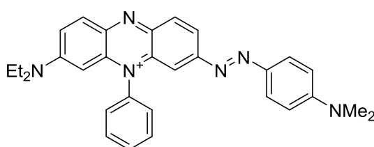
Janus Green B
