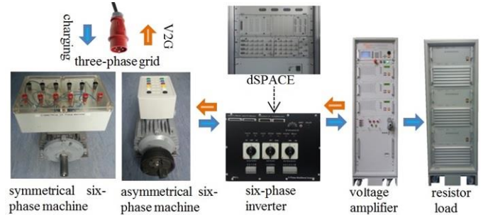
Fig. 9. Experimental rig.
