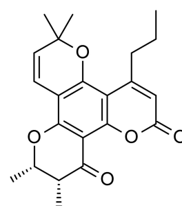
Calanolide D (7)
