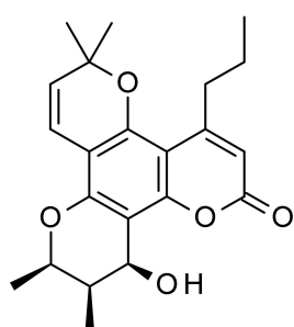
Calanolide C (6)
